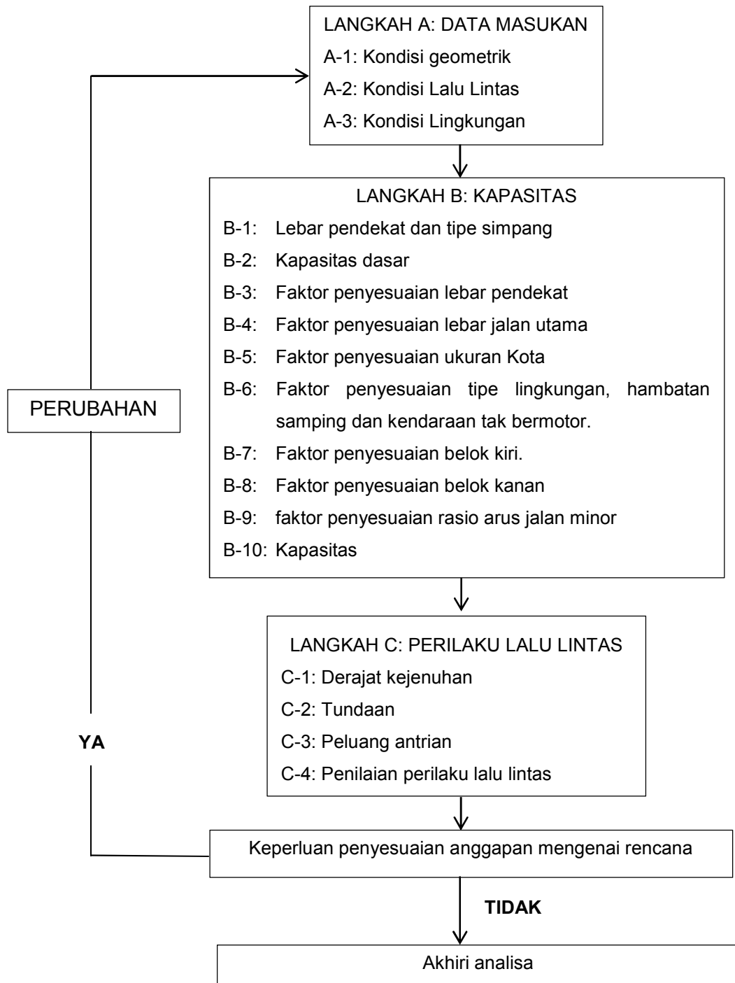
Gambar 2.6 Diagram Alir Untuk Analisis Kinerja Simpang Tak bersinyal
