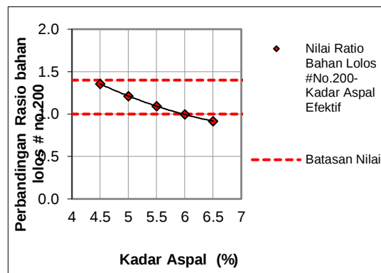
Gambar 2.9 Grafik Rasio Partikel
