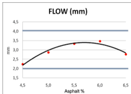
Gambar 2.5 Grafik Flow
