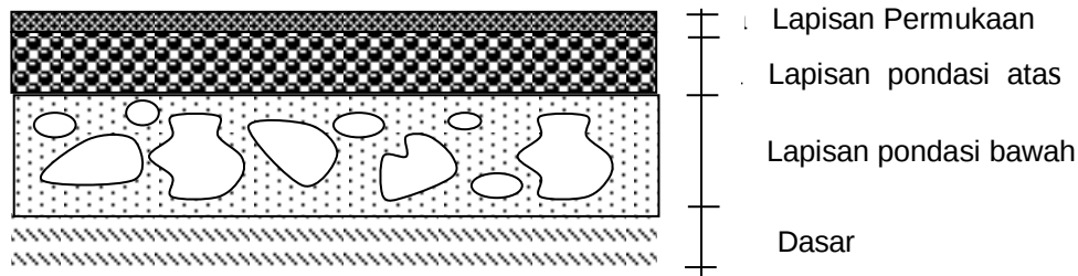
Gambar 2.1 : Susunan Perkerasan Jalan
