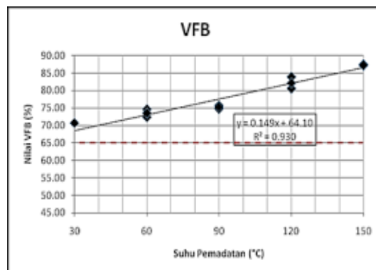
Gambar 2.8 Grafik VFB
