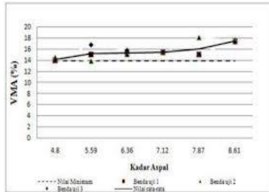
Gambar 2.6 Grafik VIM
