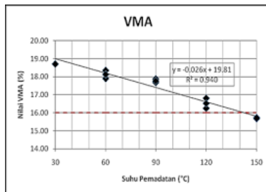
Gambar 2.7 Grafik VMA
