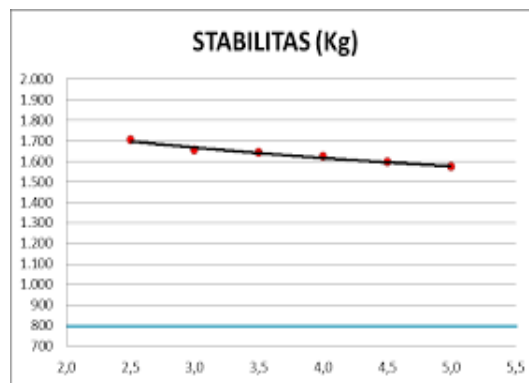
Gambar 2.4 Grafik Stabilitas
