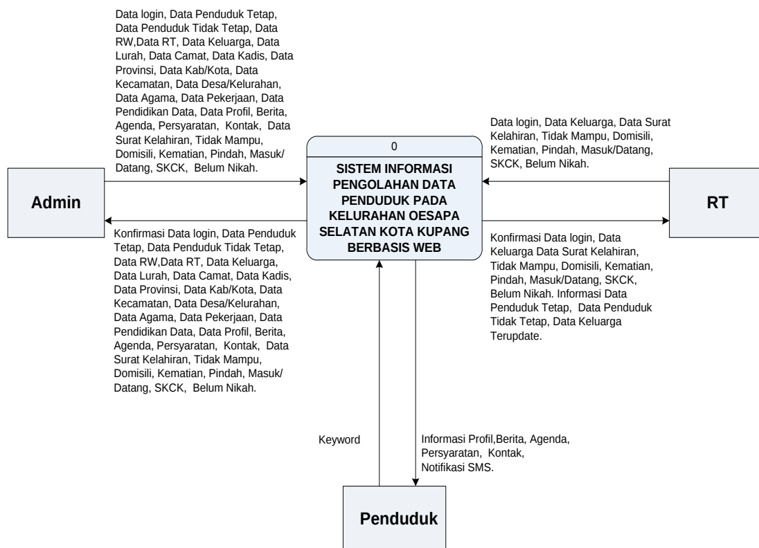
Gambar 3.2 Diagram Konteks
