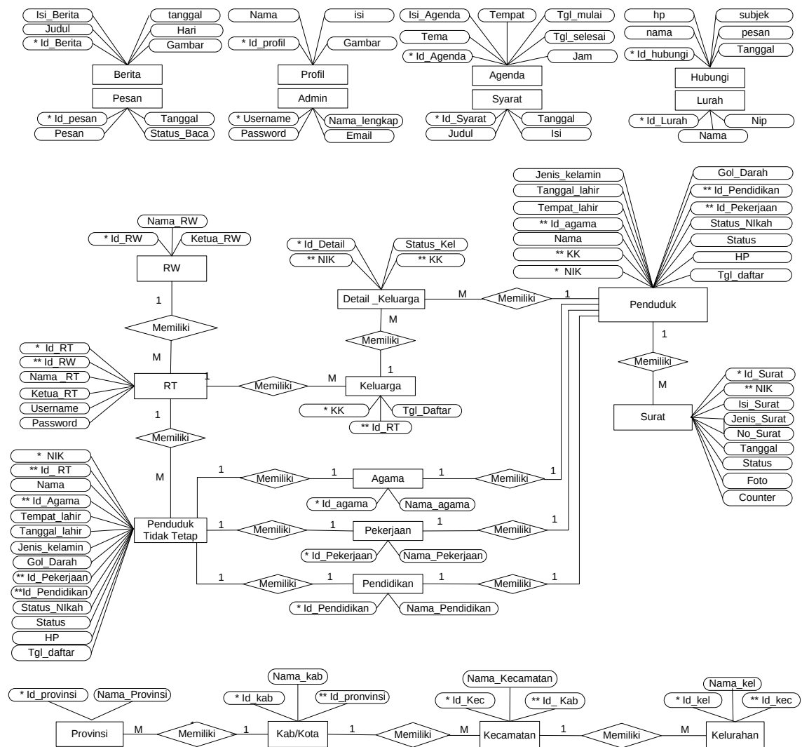
Gambar 3.4 ERD
